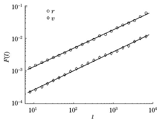
图10 收益率波动率的降趋脉动函数的示意图
