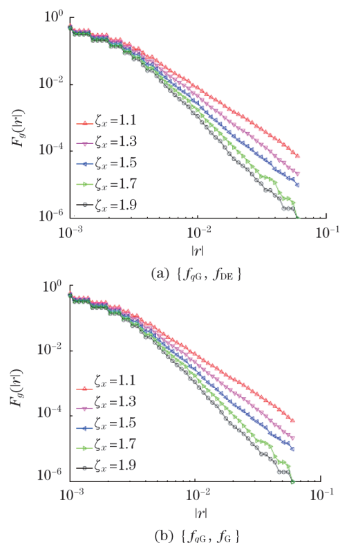
图9 \{f_{qG}, f_{DE}\} 和 \{f_{qG}, f_G\} 组合下绝对值收益率 |r| 的互补累积分布函数图
