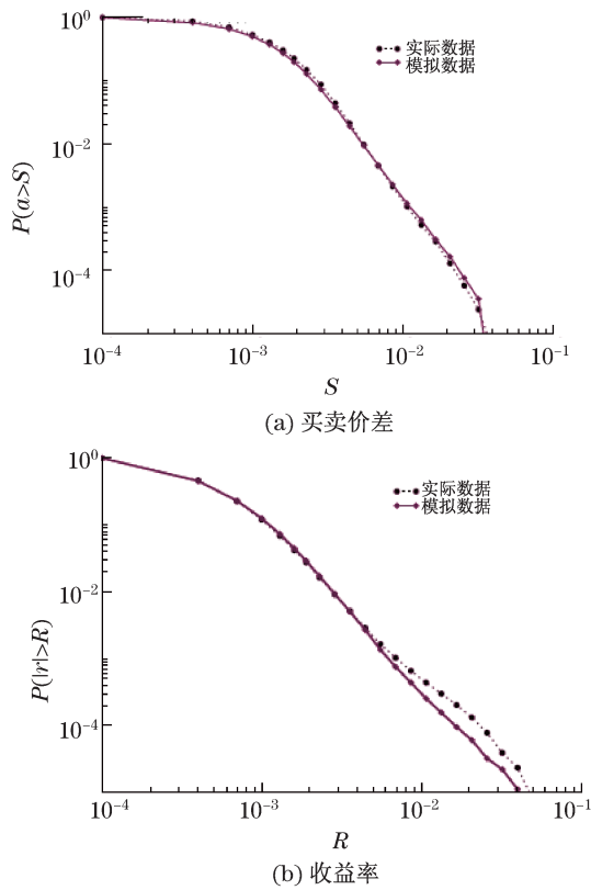
图4 买卖价差和收益率互补累积分布函数的示意图
