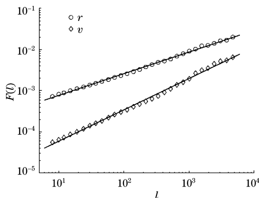
图 13 修正的 MF 模型生成的收益率、波动率的降趋脉动函数的示意图
