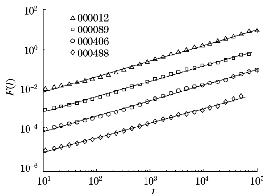
图 11 4 只股票相对价格时间序列的降趋脉动函数的示意图
