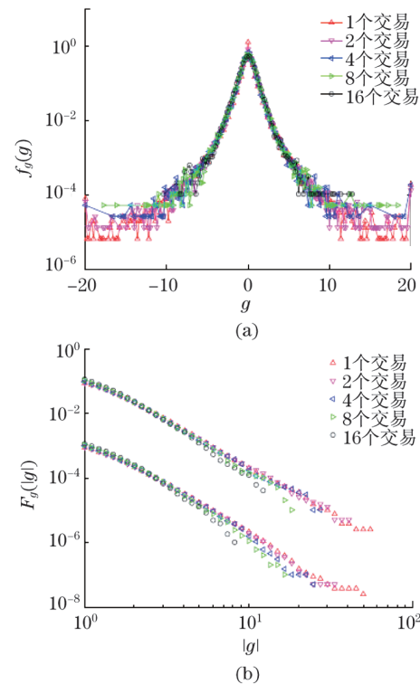
图 6 \Delta t = 1, 2, 4, 8, 16 时收益率的概率密度函数图和互补累积分布函数图
