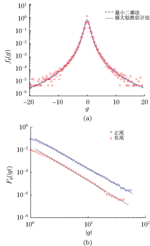
图5 \Delta t = 1 时收益率的概率密度函数和互补累积分布函数图
