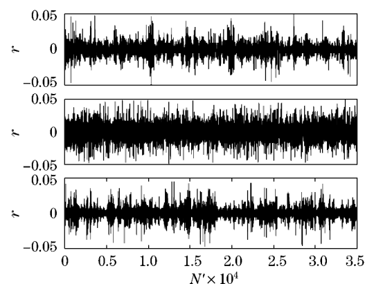
图 12 收益率片段(股票 000012(上),原始 MF 模型(中),修正的 MF 模型(下))
