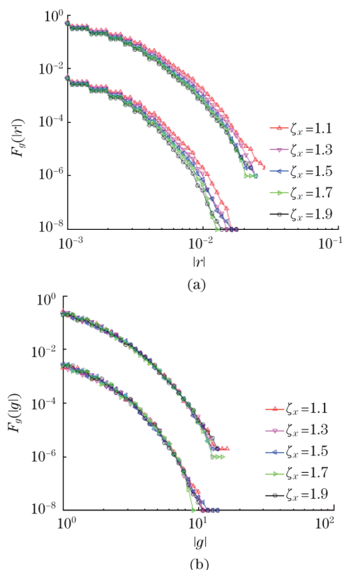
图8 两种组合下绝对值收益率 |r| 和标准化后绝对值收益率 |g| 的累积分布函数图
