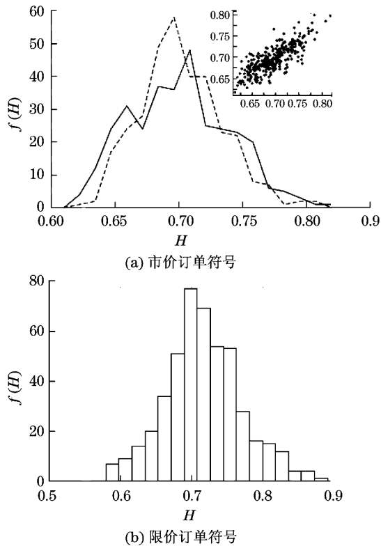
图1 市价订单符号和限价订单符号赫斯特指数 H 的分布图
