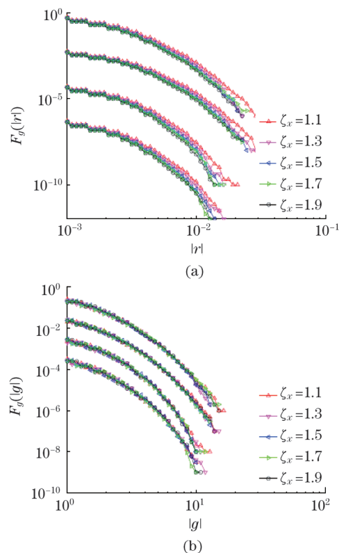
图7 4种组合下绝对值收益率 |r| 和标准化后收益率 |g| 的累积分布函数的示意图
