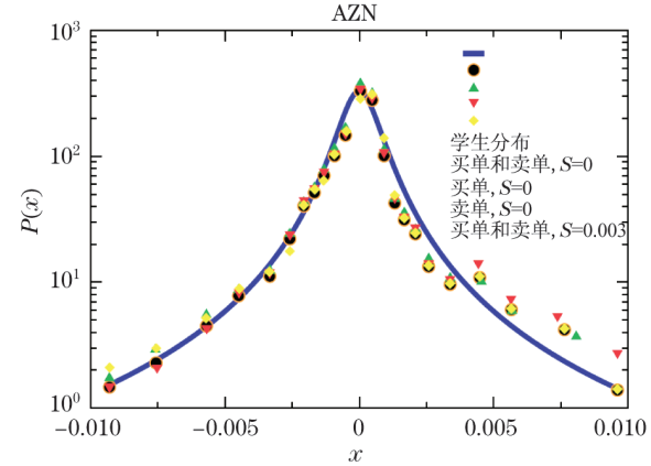
图2 股票 AZN 相对价格 x 的概率密度函数 P(x) 的示意图 Fig.2 Plot of the probability density function P(x) of relative prices x
